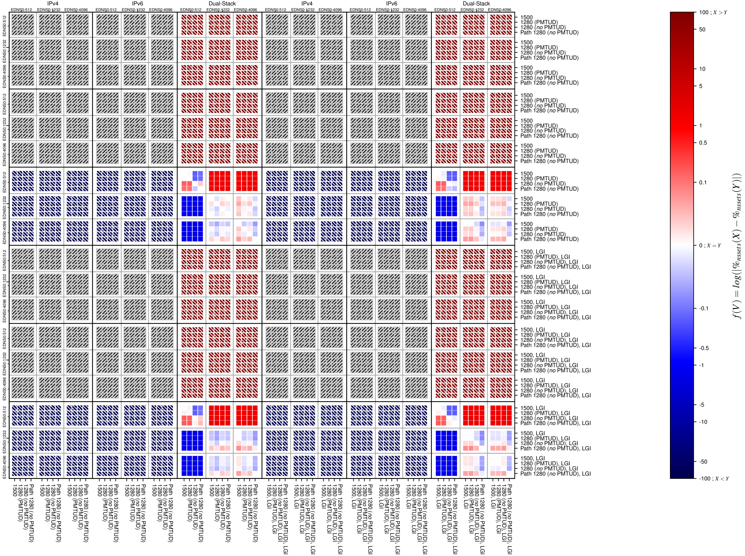
no_dnssec-v4-UDP_TCP_afc_count
