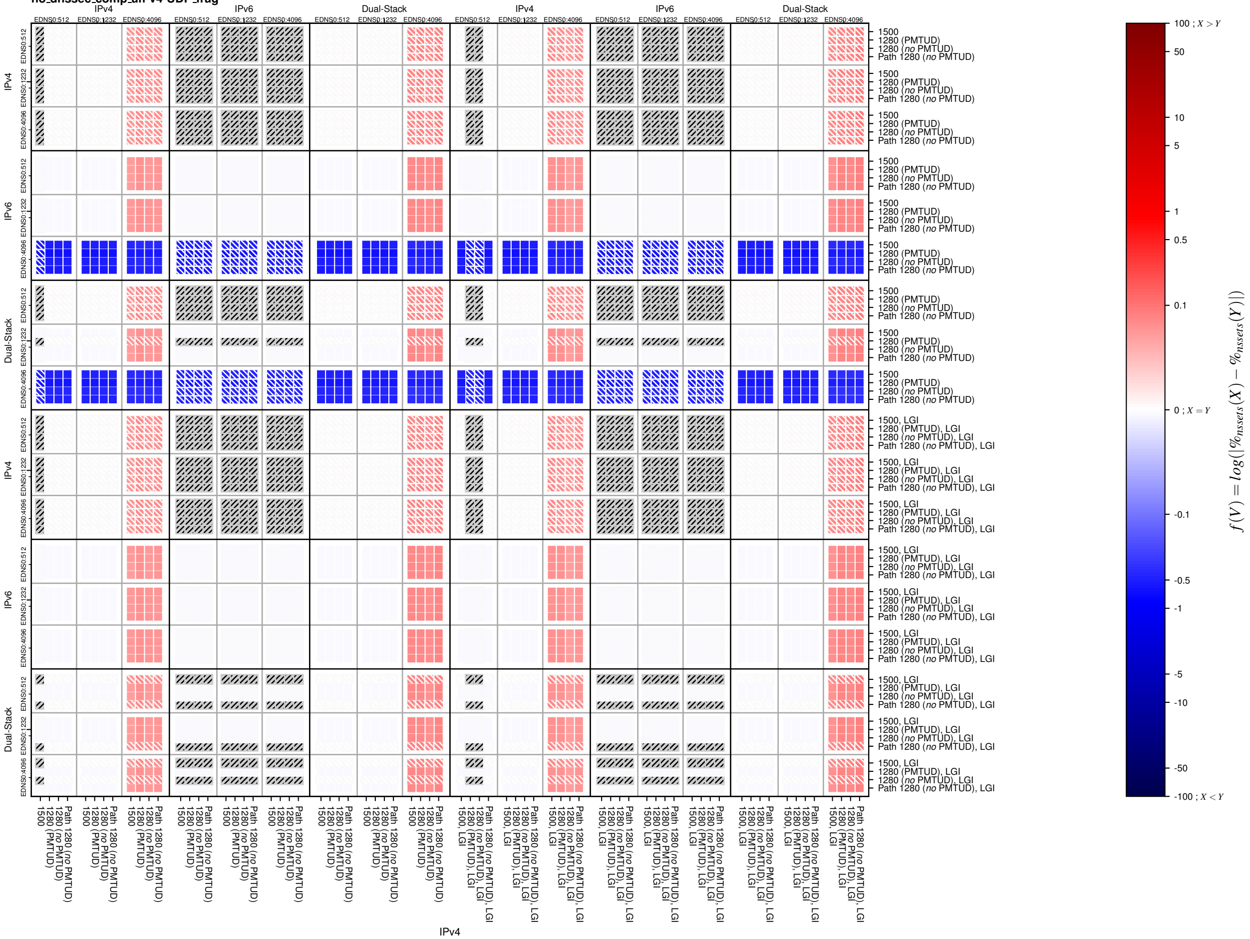
no_dnssec_comp_afv-v4-UDP_frag
