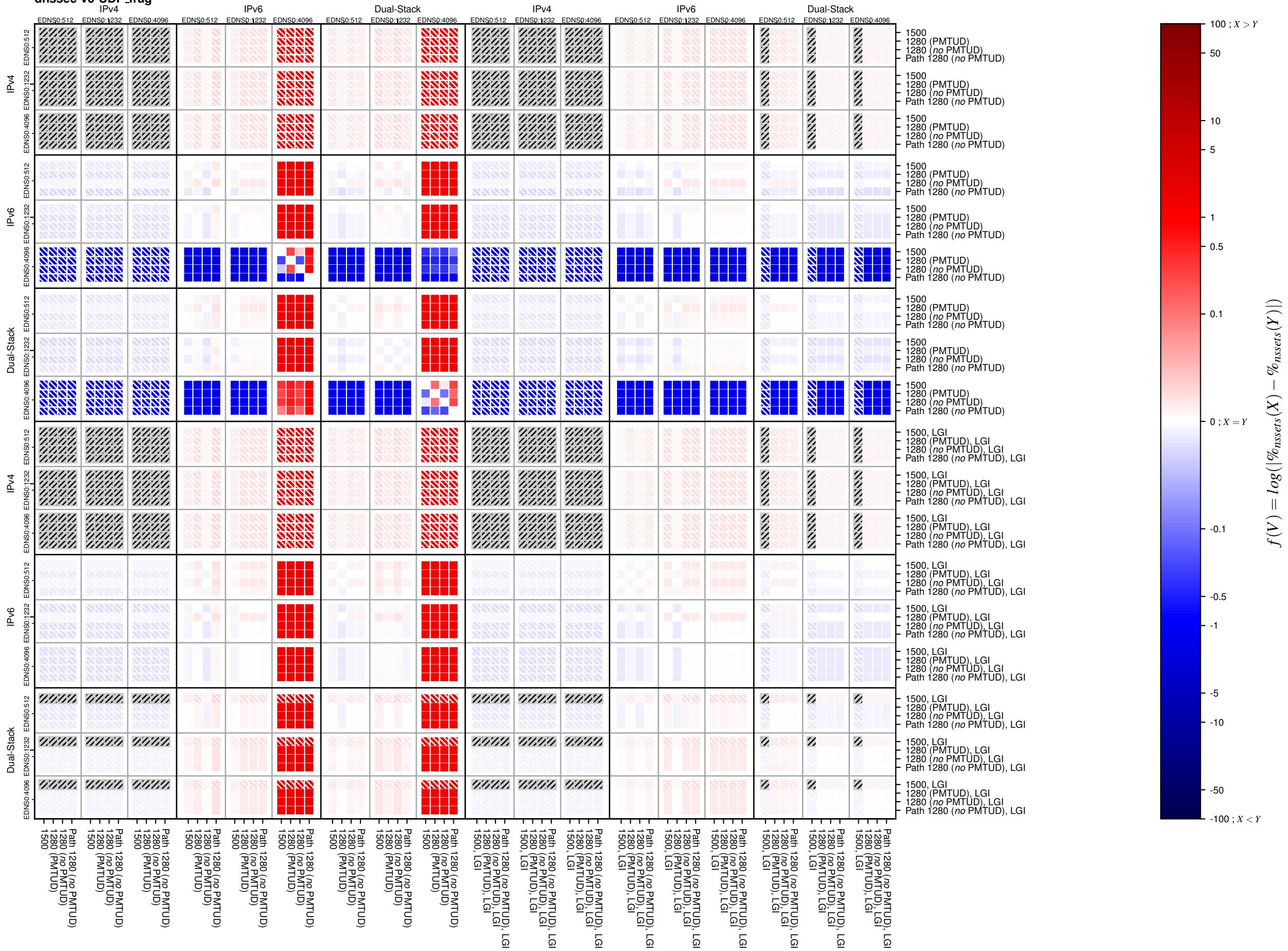
dnssec-v6-UDP_frag
