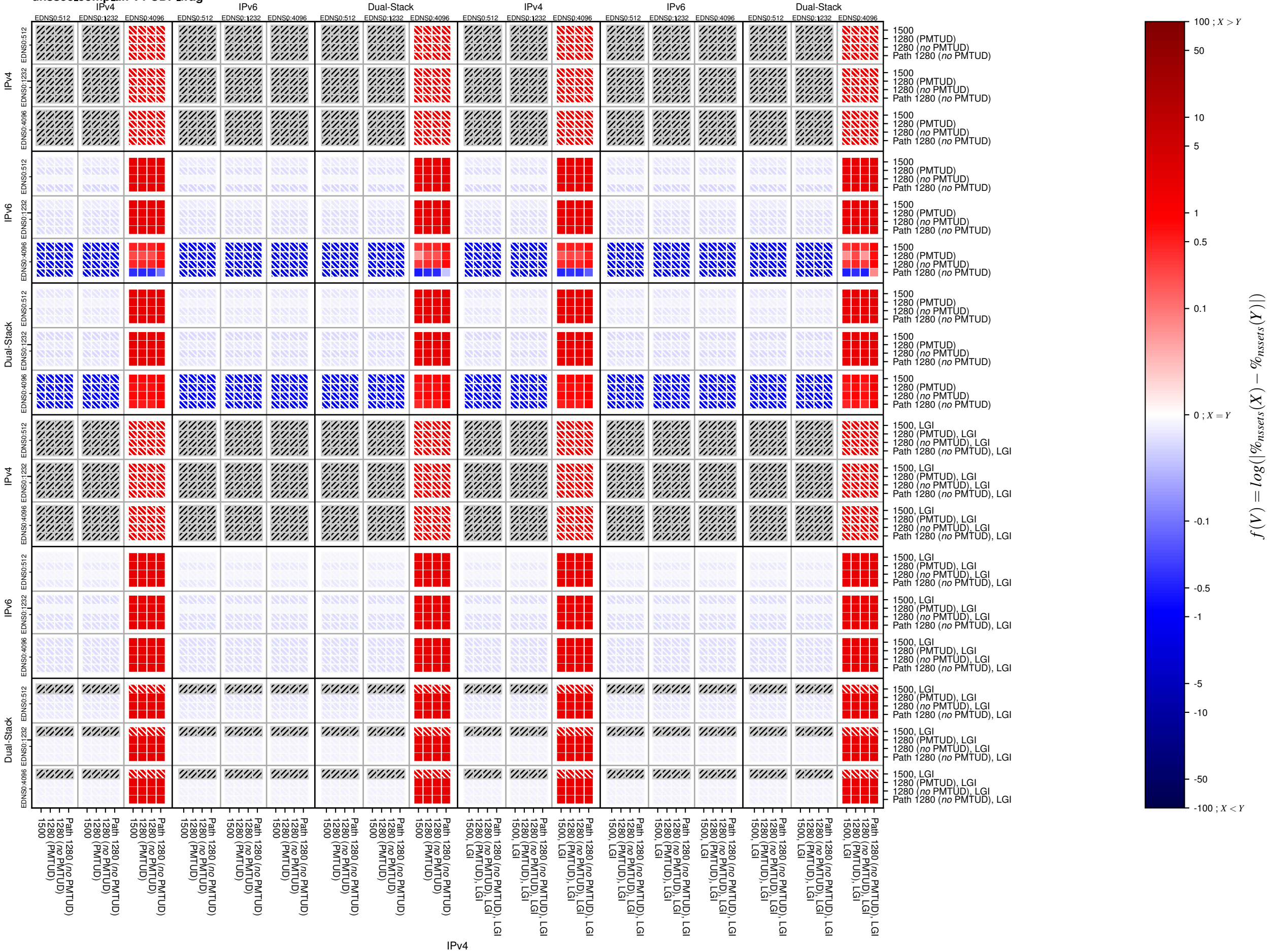
dnssec_comp_afi-v4-UDP_frag
