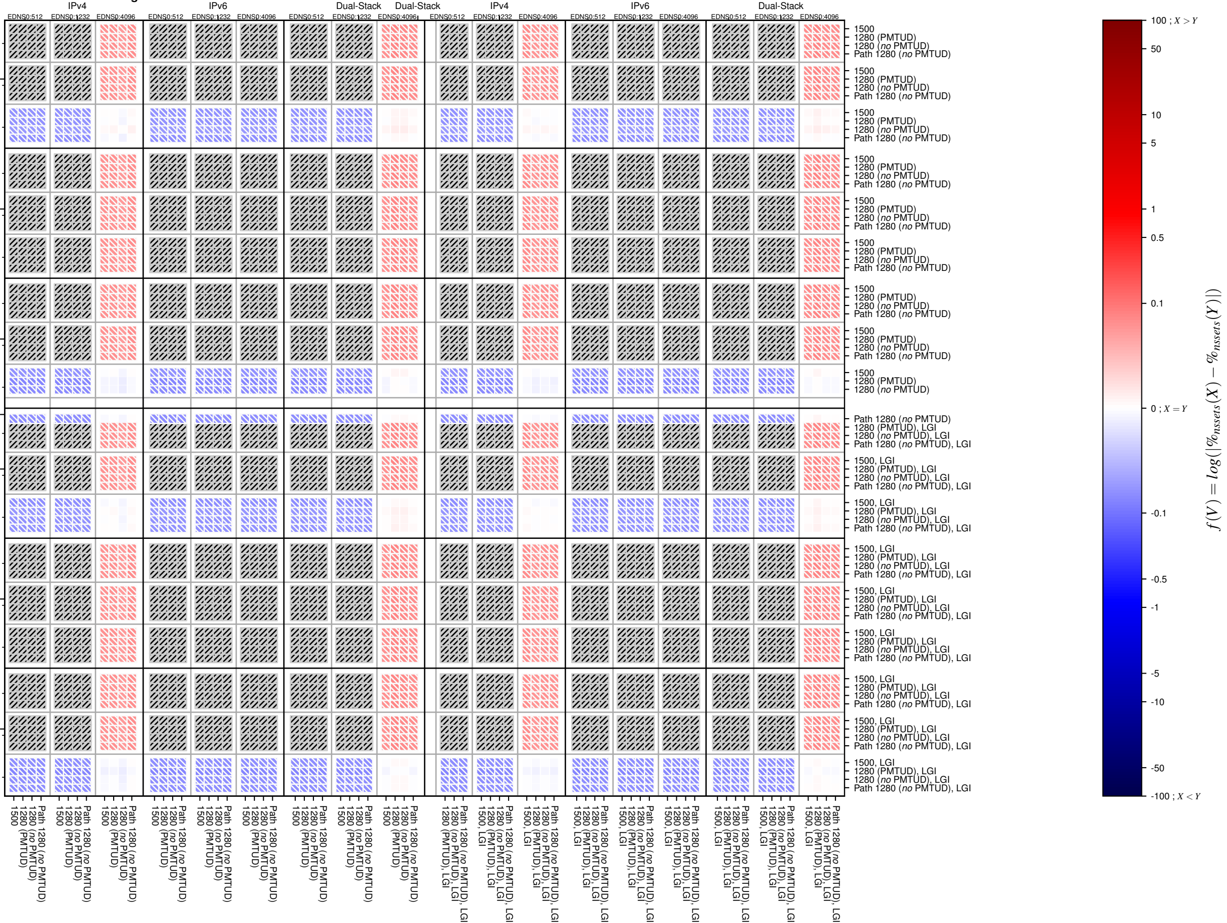
no_dnssec-v4-UDP_frag
