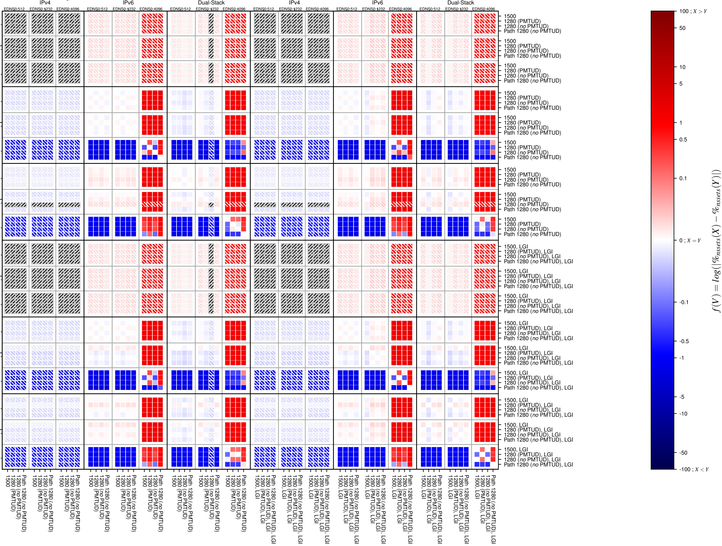
dnssec-v6-UDP_frag
