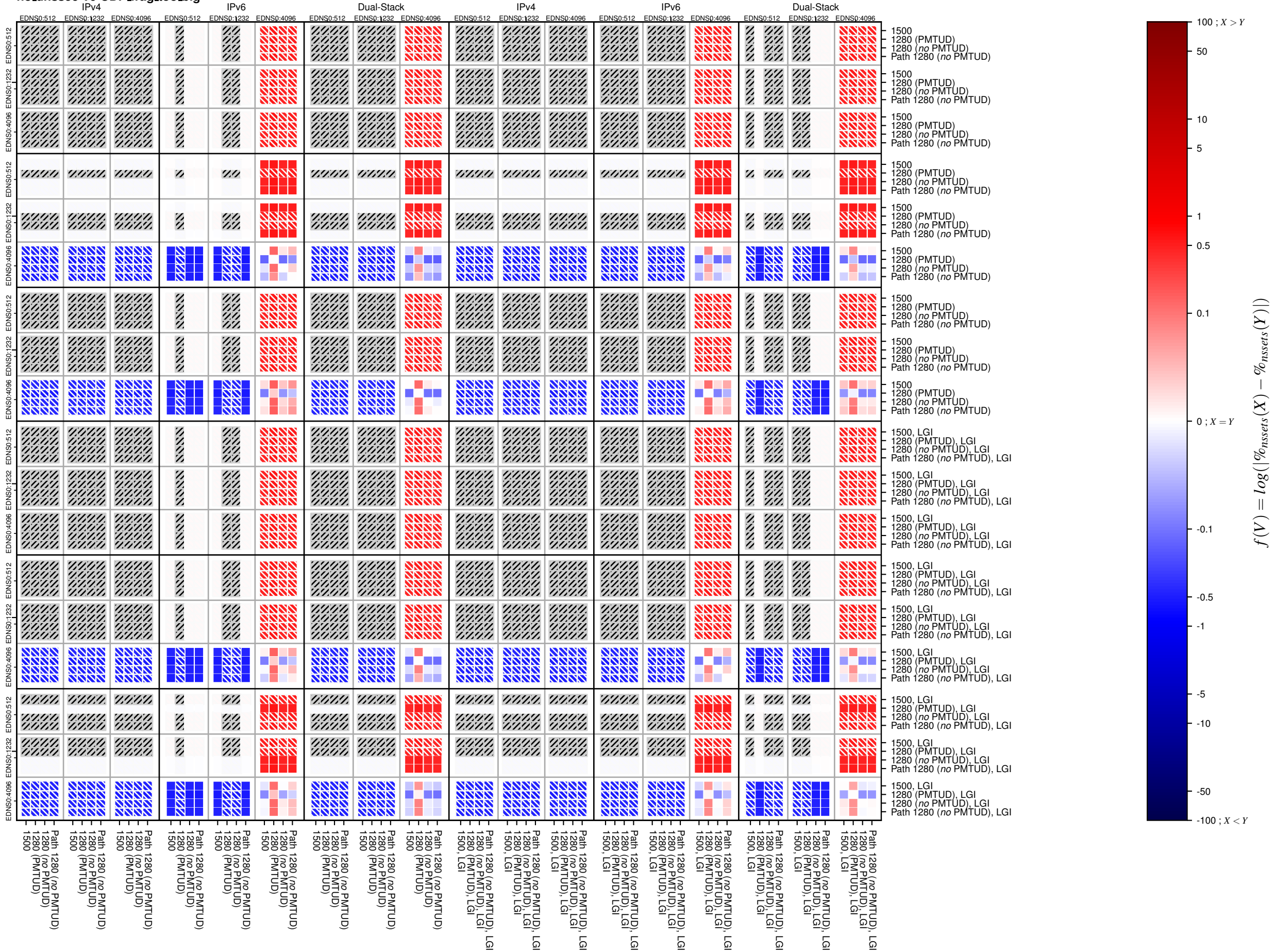
no_dnssec-v6-UDP_frag_too_big
