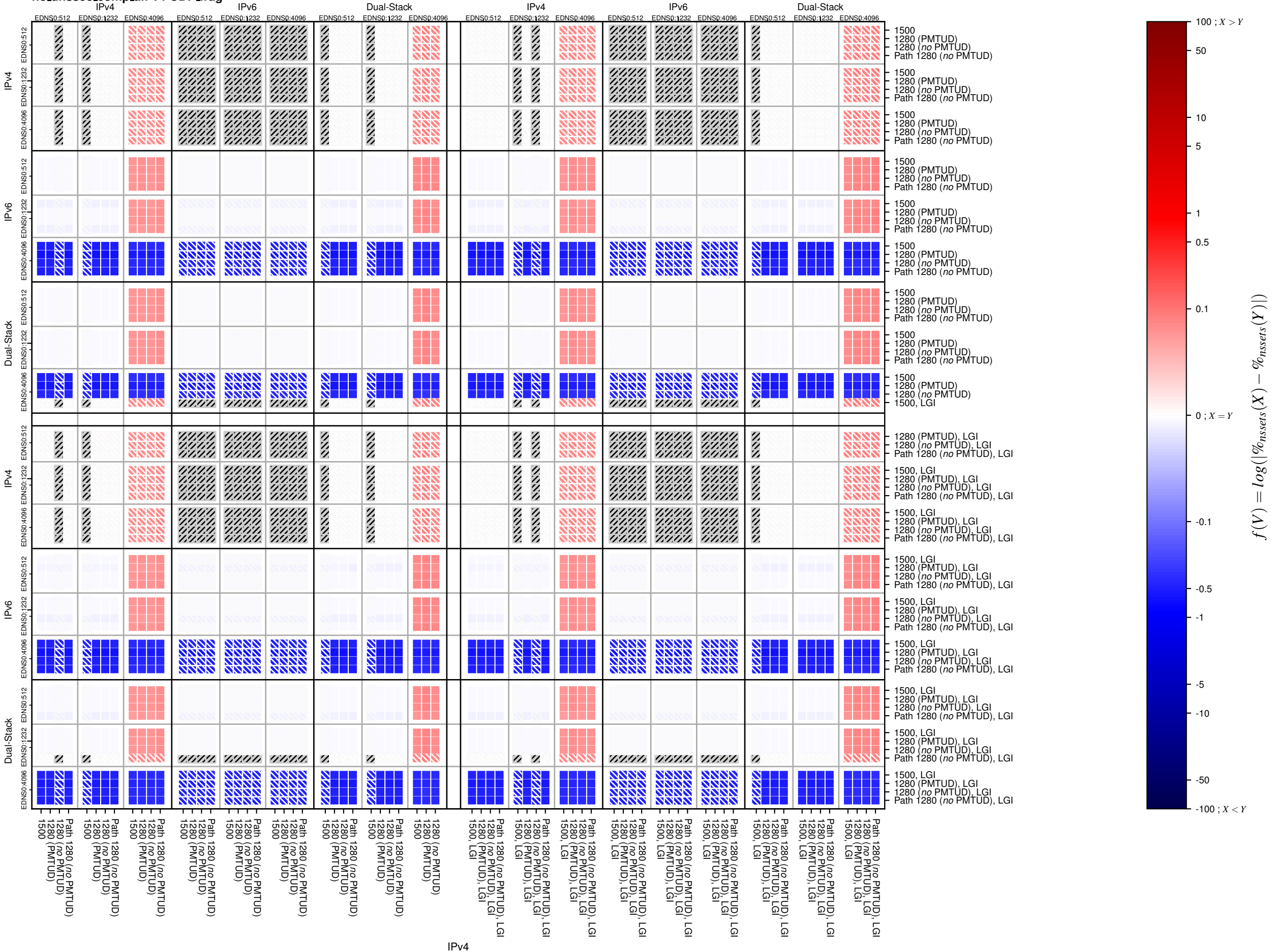
no_dnssec_comp_afi-v4-UDP_frag
